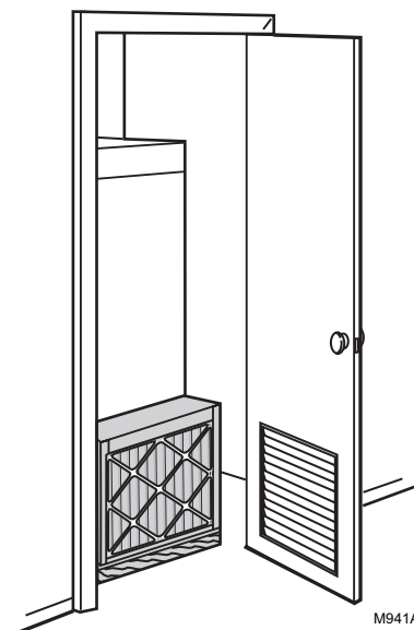
Fig. 3. Appareil de chauffage superposé avec installation dans un placard. L'épurateur d'air à fibres se monter verticalement sur l'appareil de chauffage entre ce dernier et l'ouverture de l'air de retour à volets de la porte du placard.
