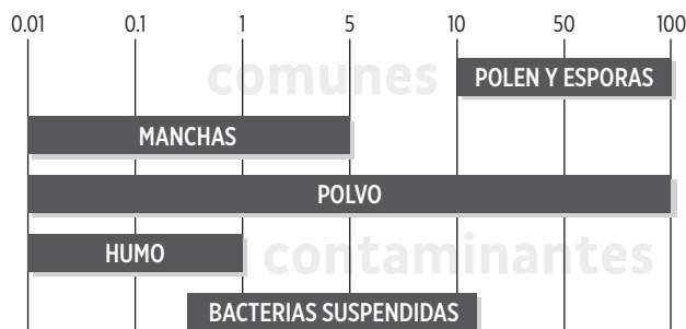
FIGURA 2 – CONTAMINANTES COMUNES
