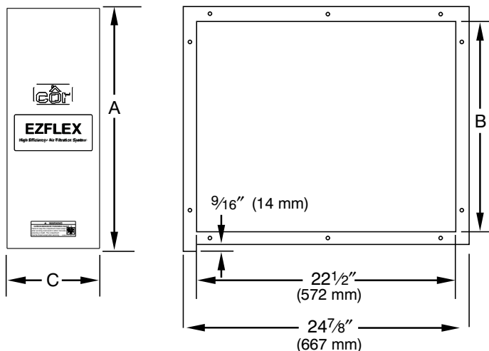
Fig. 5 – EZXCABCR Dimensions
