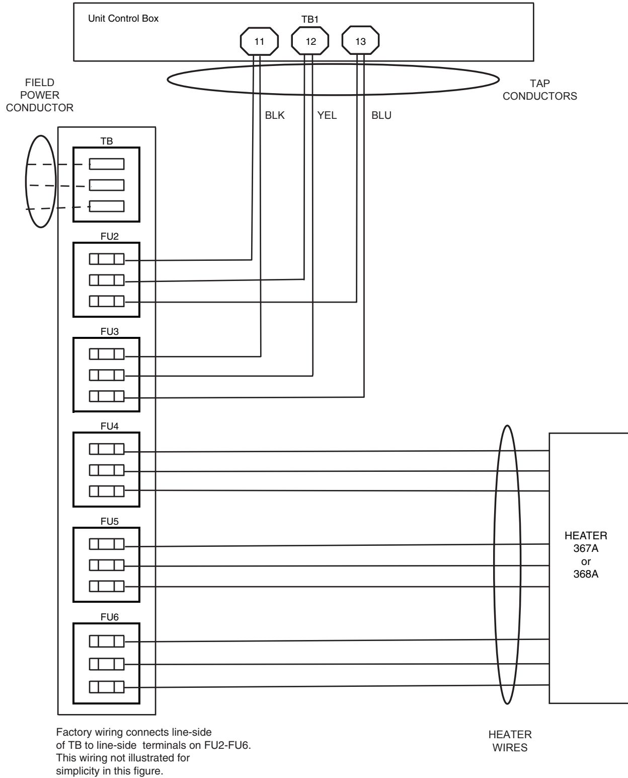
Fig. AV — Heat Pump Single Point Box CRSINGLE054A00 (HP-1, Size 14; HP-2, Size 12)
