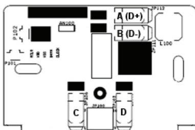
Fig. 3 – Backplate
