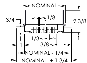
LTM 1/3 0°
