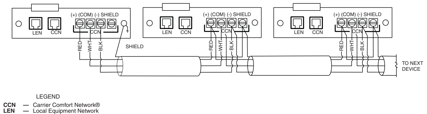
Fig. 33 — TB3 — CCN Wiring
