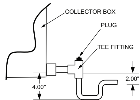
Fig. 135 — Condensate Drain
