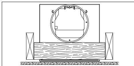
Supports retournés et fixés de part et d'autre de la sortie du boîtier.
