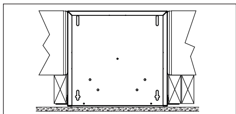
Supports fixés de part et d'autre de la sortie du boîtier.
