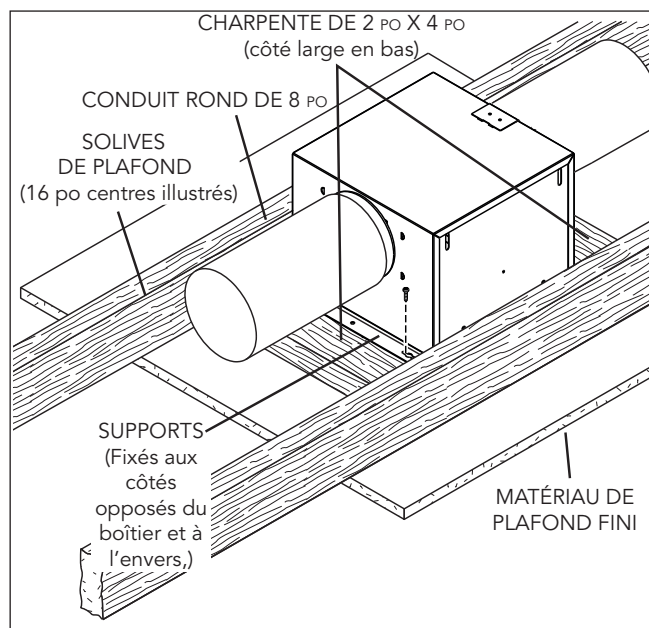
Appareil installé dans un bâtiment déjà construit .
