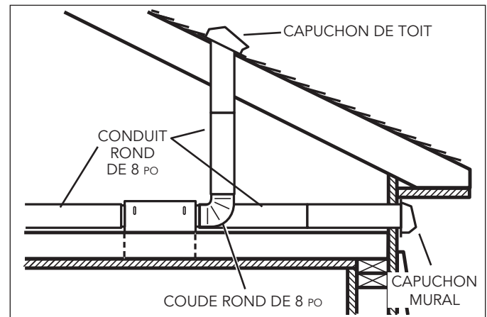
Deux manières de raccorder les conduits.
