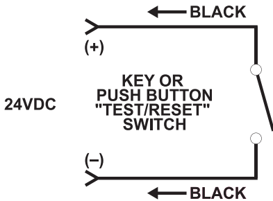
TEST/RESET
