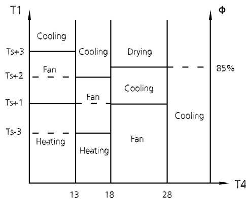
Fig. 8 – Auto Mode
