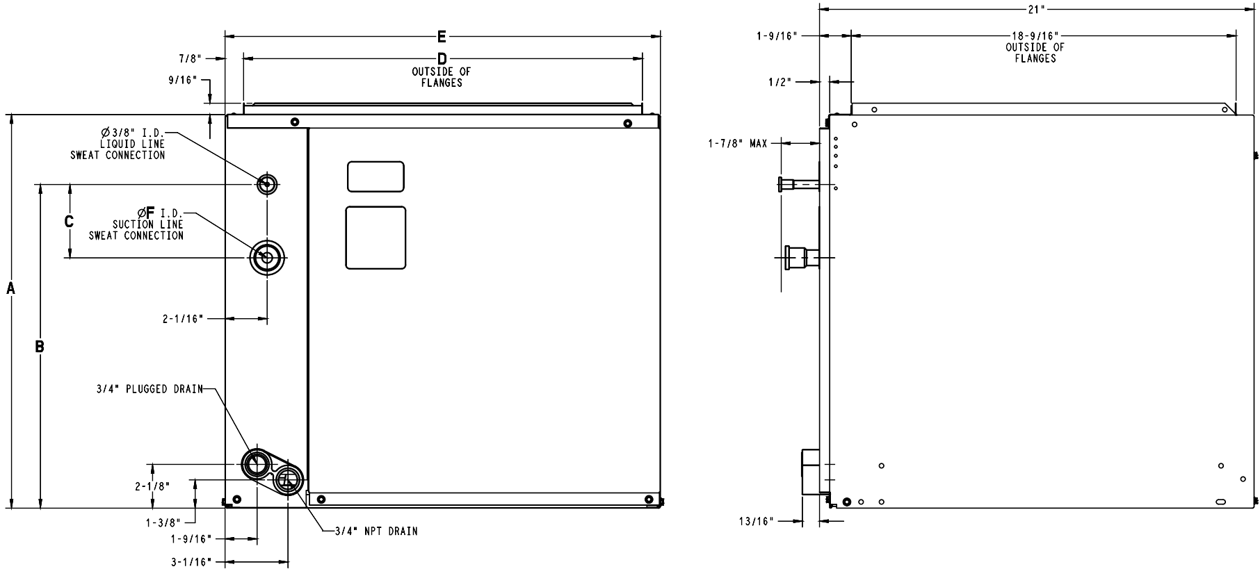
Fig. 2 – Dimensions (English)
