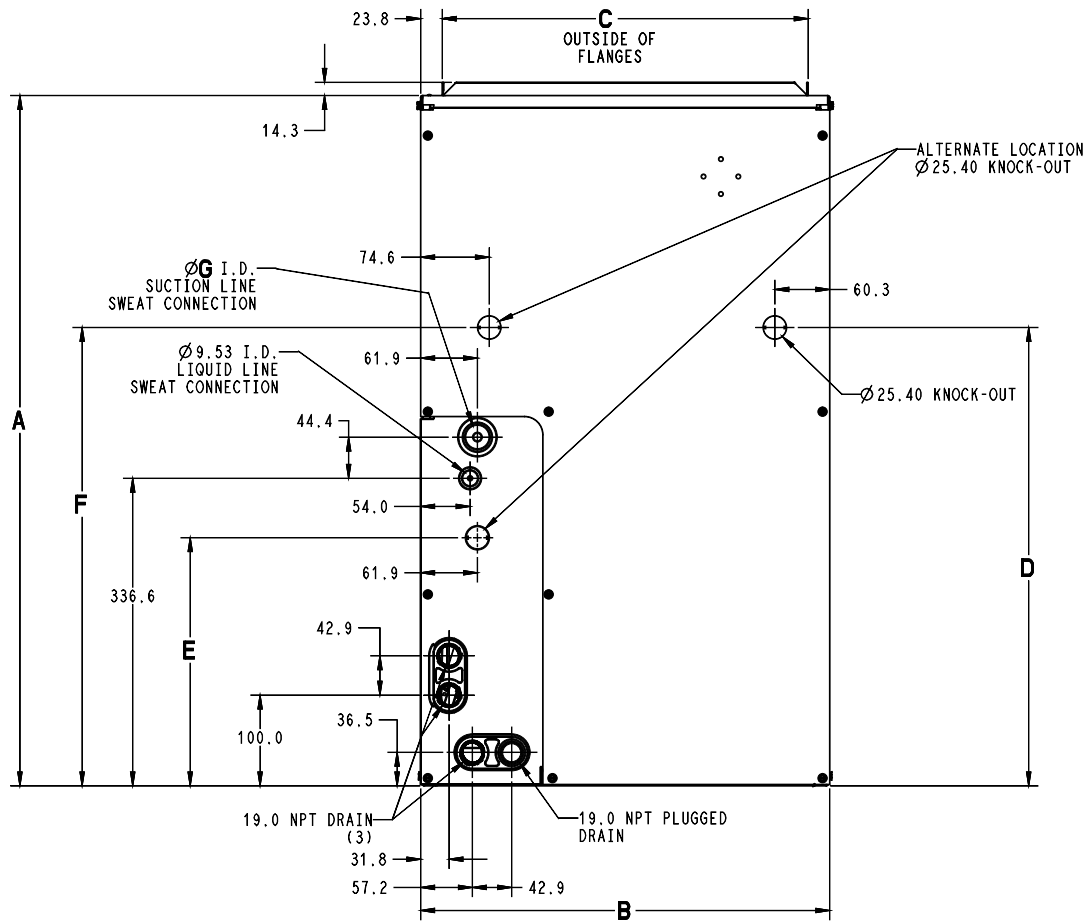
Fig. 3 – Dimensions (Metric)
