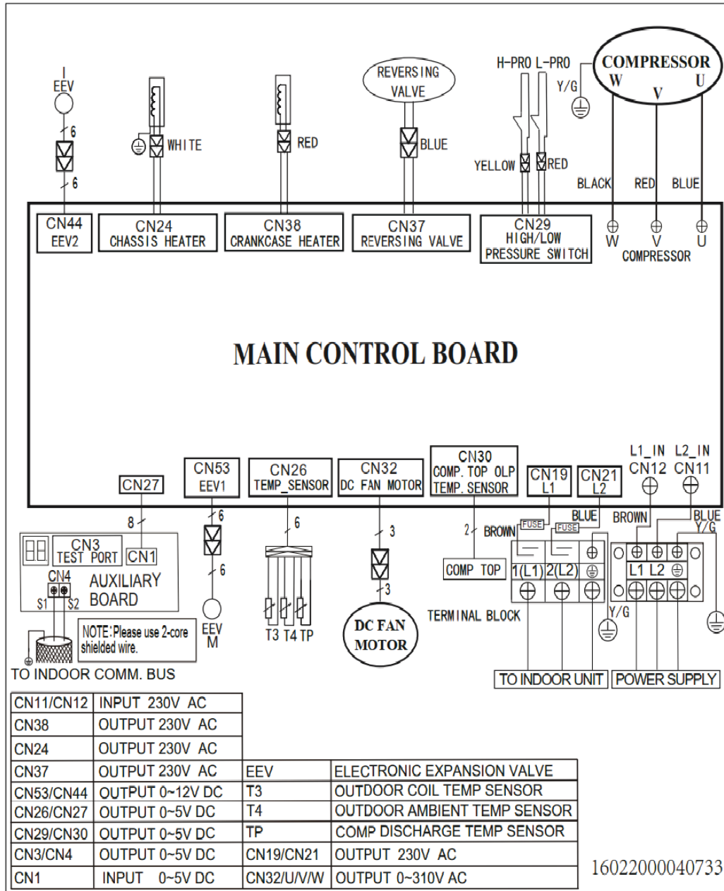
Fig. 7 – 36K Wiring Diagram
