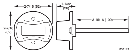
Fig. 1. Dimensions du C7735A en po (mm).
