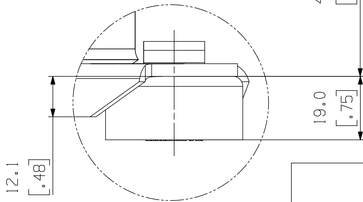
DETAIL Y SCALE 3:2
