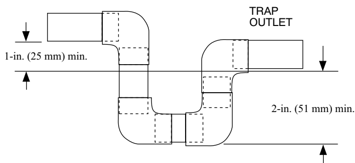
Fig. 7 – Condensate Trap
