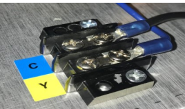
24 volt connection
