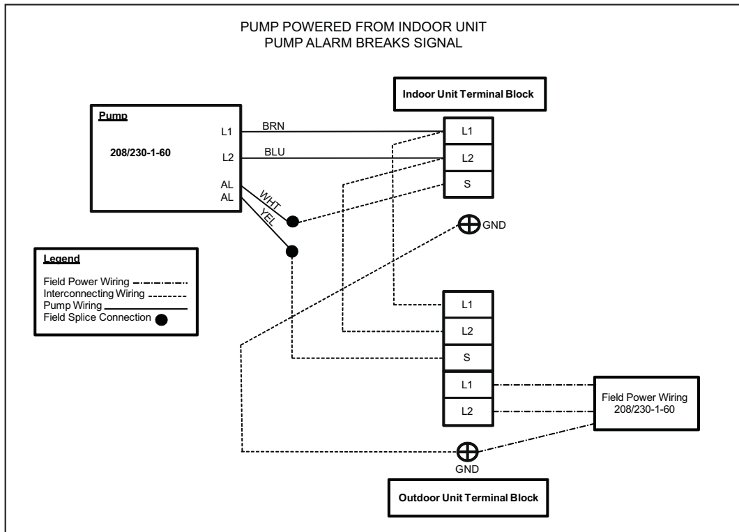
Fig. 15 – (208/230-1-60) WIRING SCHEMATIC
