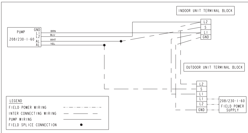
Fig. 19 – (208/230-1-60) WIRING SCHEMATIC
