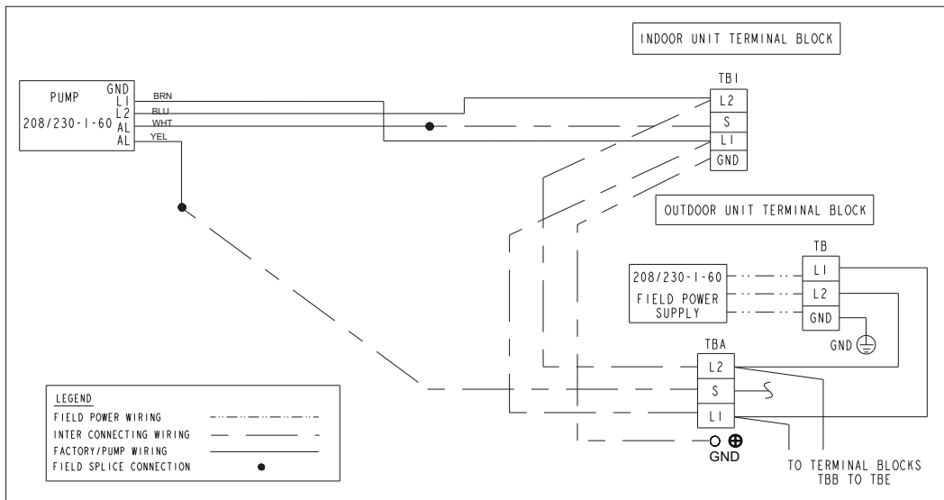
Fig. 20 – (208/230-1-60) WIRING SCHEMATIC
