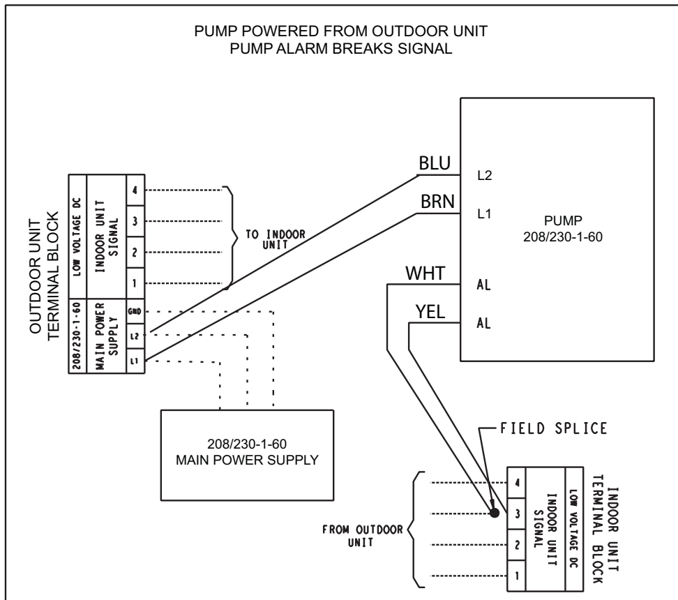
Fig. 10 – (208/230-1-60) WIRING SCHEMATIC
