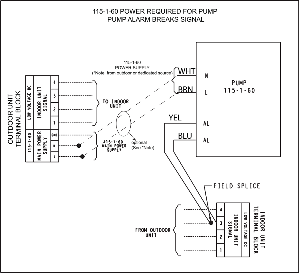
Fig. 8 – (115-1-60) WIRING SCHEMATIC
