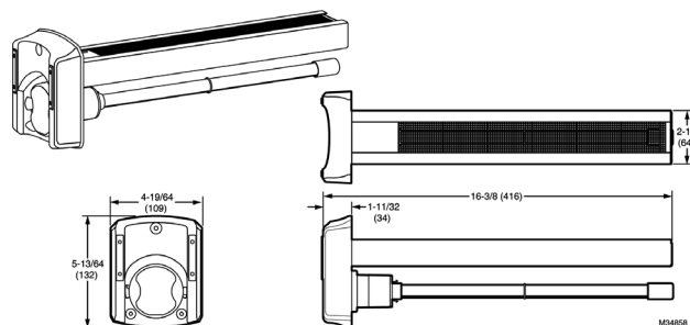
Fig. 1. Dimensiones en pulgadas (mm) del UV2400U5000.
