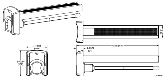
Fig. 1. UV2400U5000, Dimensions en po (mm).
