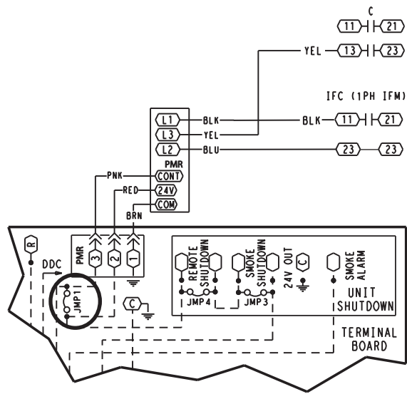
Fig. 8 - Wiring Diagram
