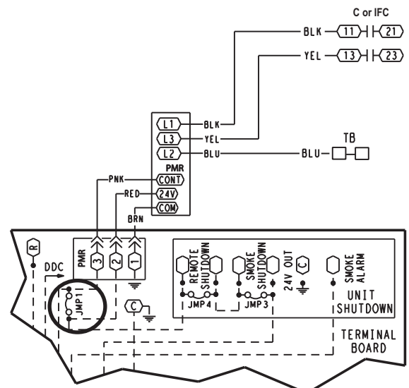
Fig. 7 - Wiring Diagram
