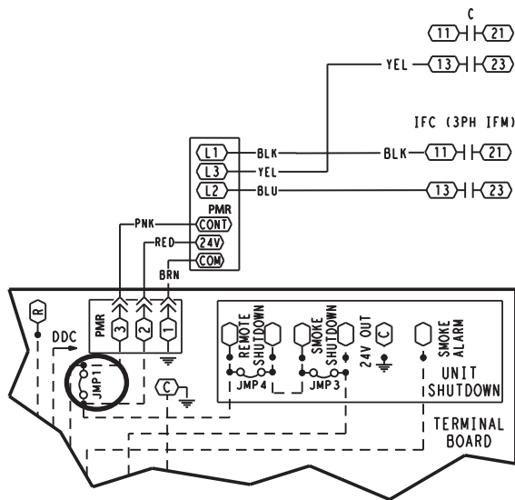
Fig. 6 - Wiring Diagram
