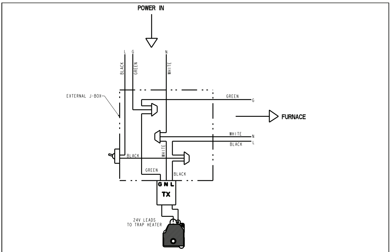
Fig. 1 - Wiring Schematic
