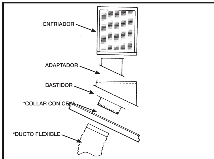
SALIDA INFERIOR
