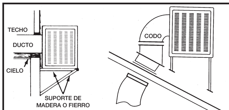
DESCARGA LATERAL
