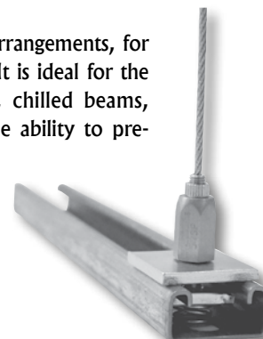
3/8" Dyna-Stud
