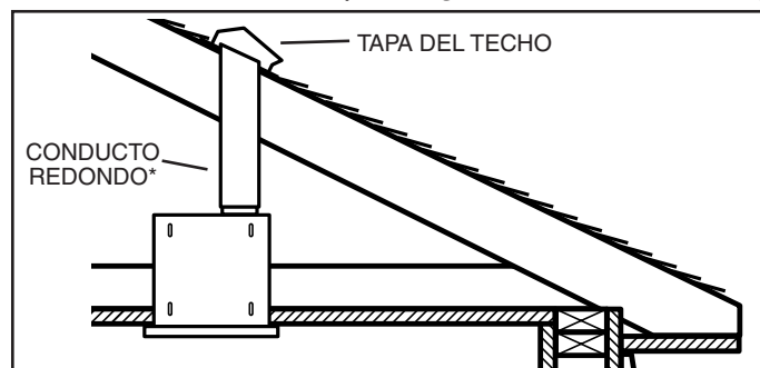
Conexión típica de los conductos al ventilador cambiado a descarga vertical.
