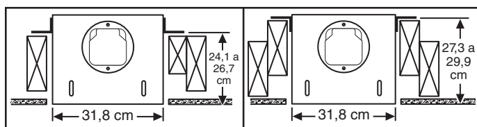
Abrazaderas de montaje montadas en la parte superior de los lados del alojamiento. (La salida queda paralela a las viguetas) (Estructura nueva o existente )
