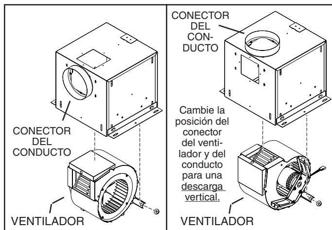
Cambie la posición del conector del ventilador y del conducto para una descarga vertical .
